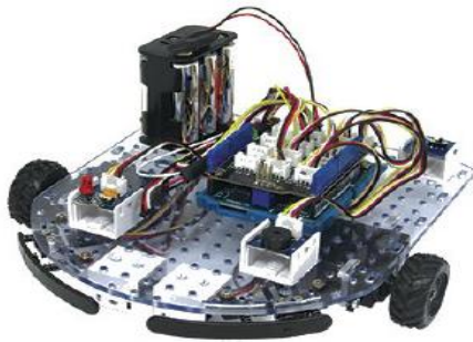
Câblage interface d'un robot
